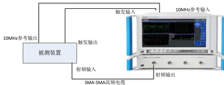
图 4.1 被测设备与基站测试仪连接图
