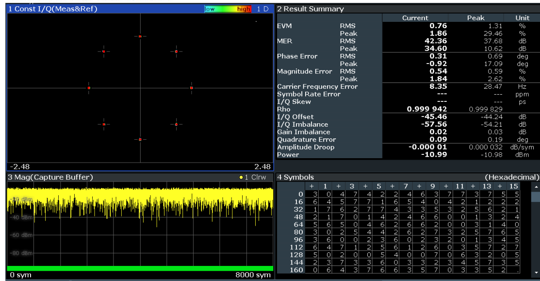
图 4.8 测试结果
