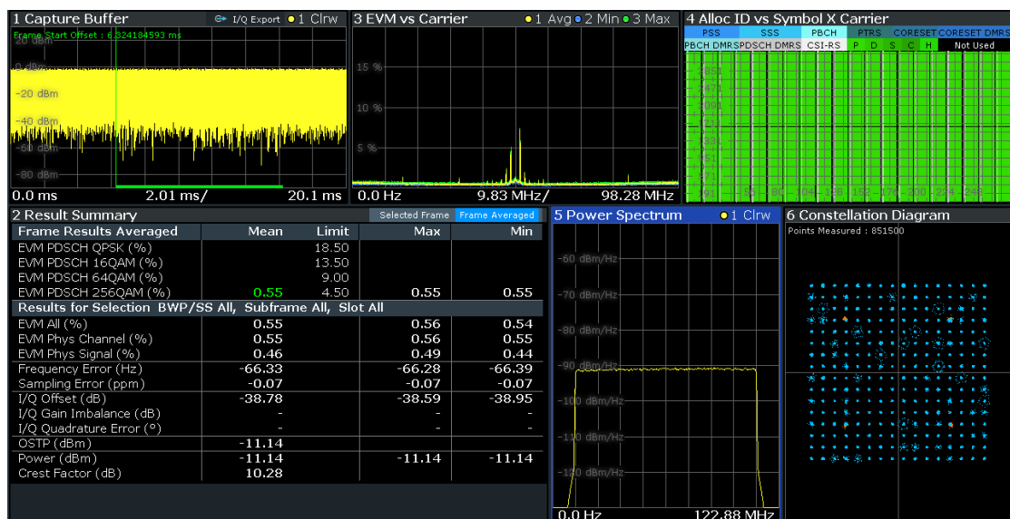
图 4.8 测试结果
