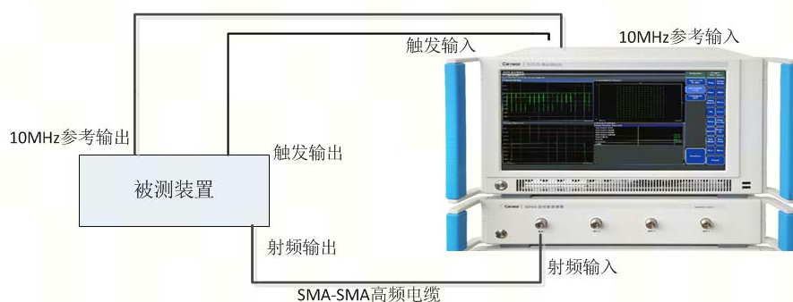
图 4.7 被测设备与基站测试仪连接图
