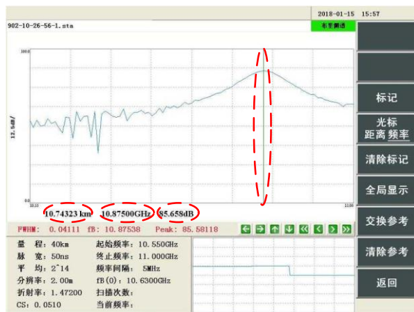
图 8-12 布里渊谱窗口
