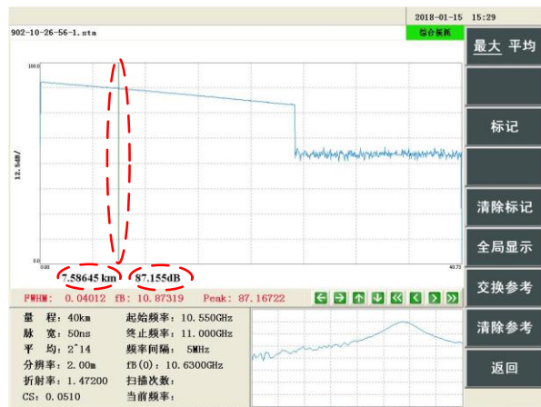
图 8-11 光纤综合损耗曲线
