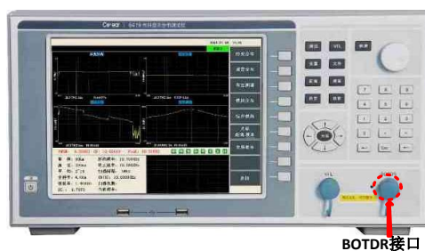
图 8-3 BOTDR 接口
