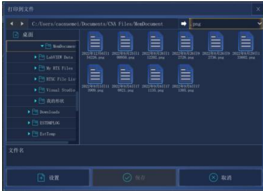
图 3.68 打印到文件
