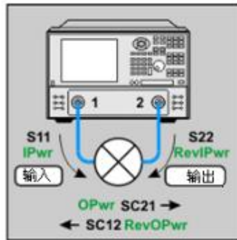
附图 6.18 测量参数示意图
