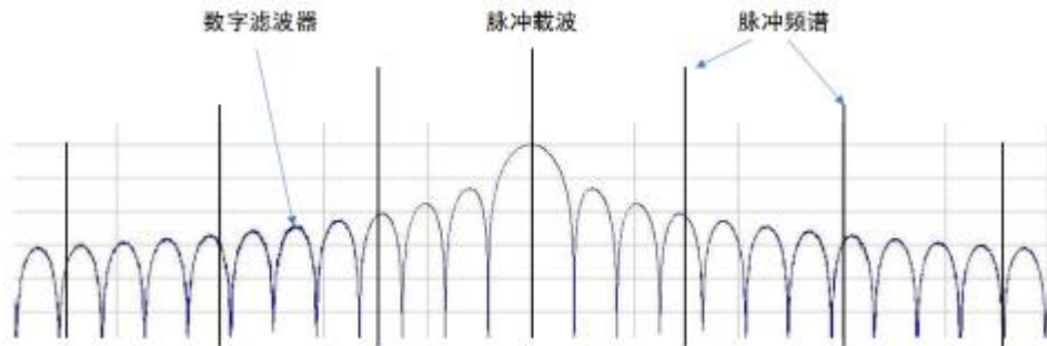
附图 4.9 中频滤波示意图
